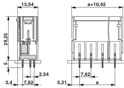
外形寸法
