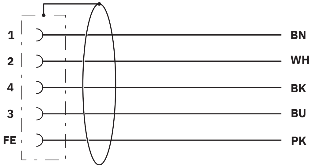
Schaltplan
