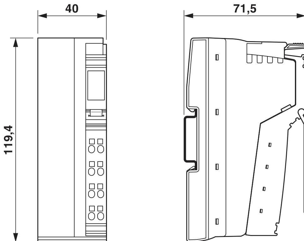
尺寸图
