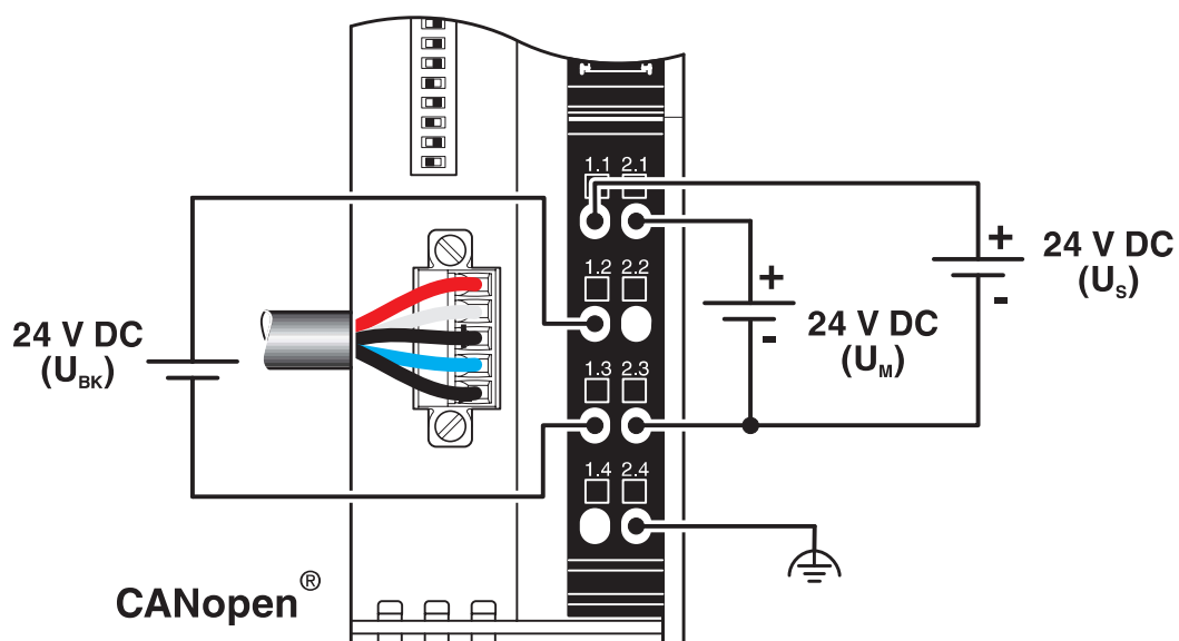
接线图
