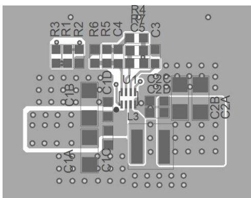
Top Layer
