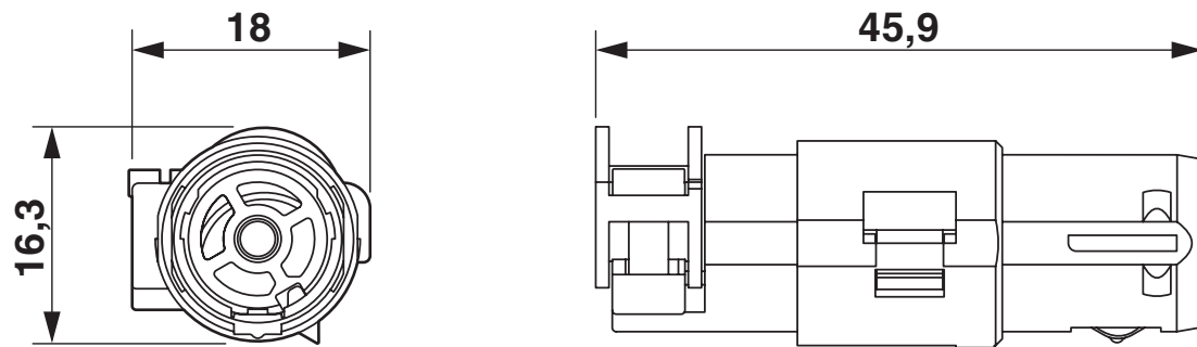
尺寸图
