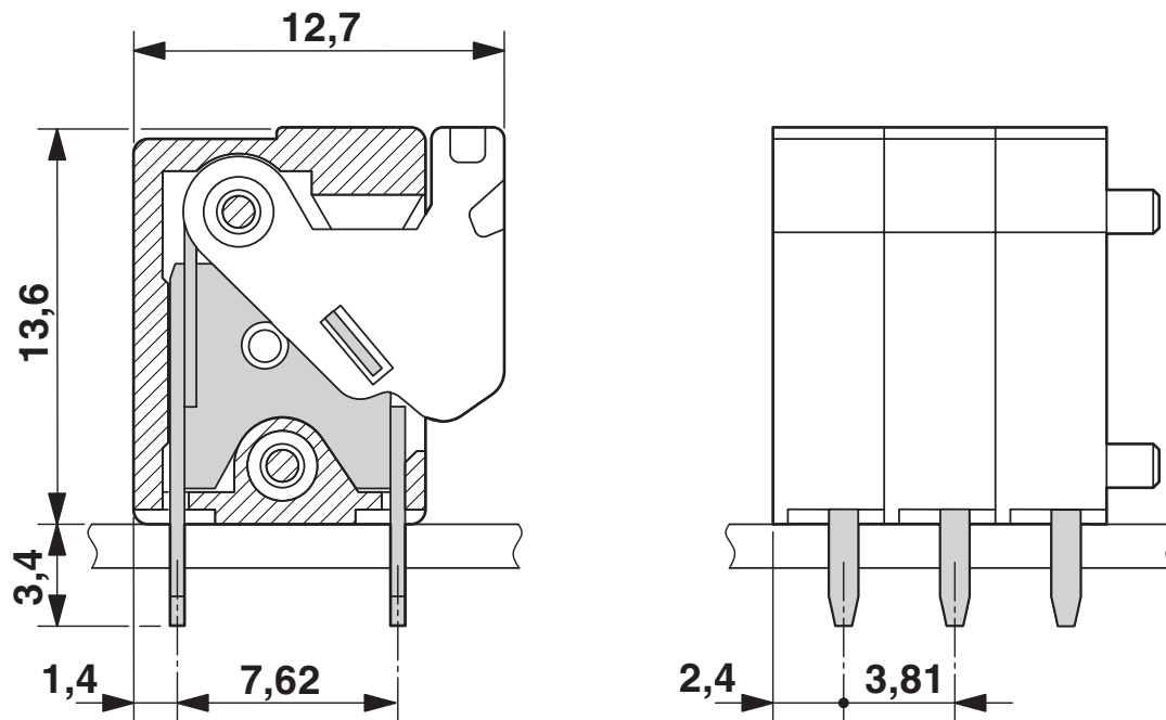
尺寸图
