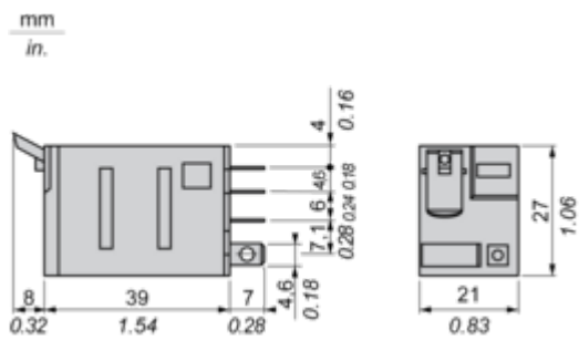
Stecker-Seitenansicht
