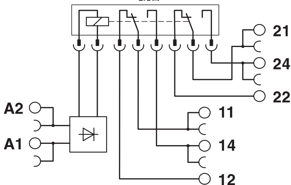
电路图
