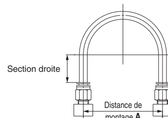
Fig. 1 : Raccordement recommandé
