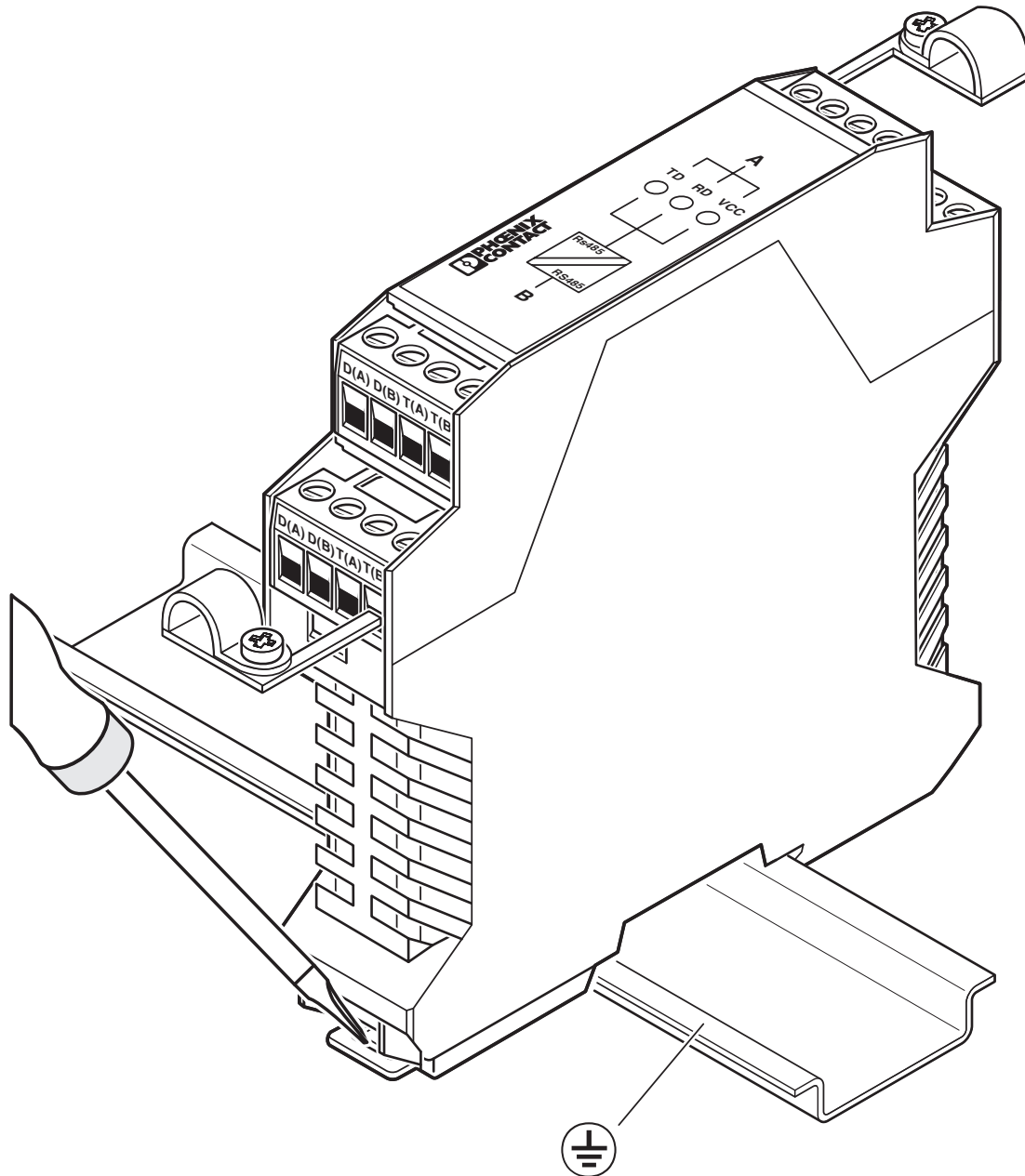
Schemazeichnung
