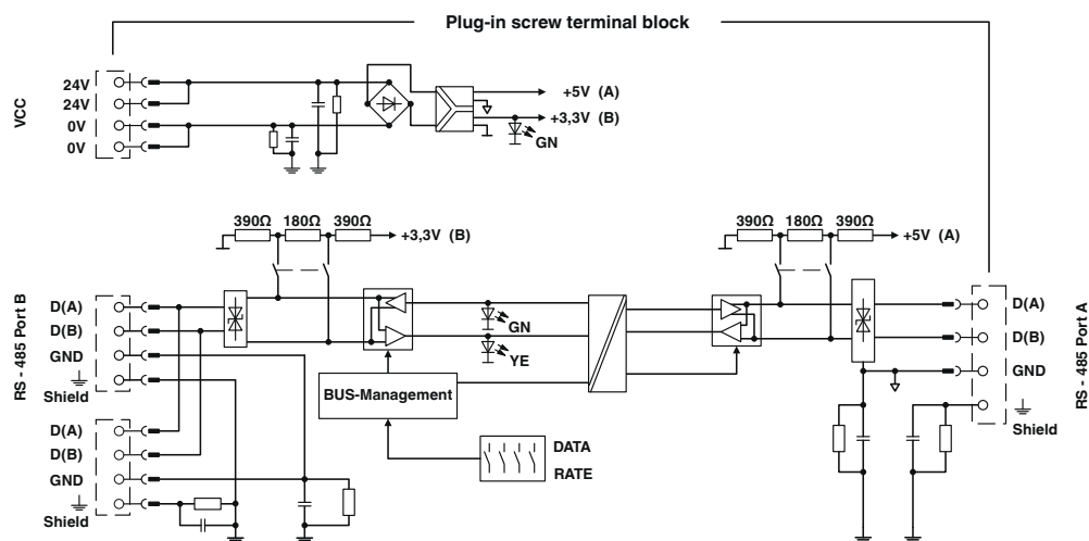
Schaltplan
