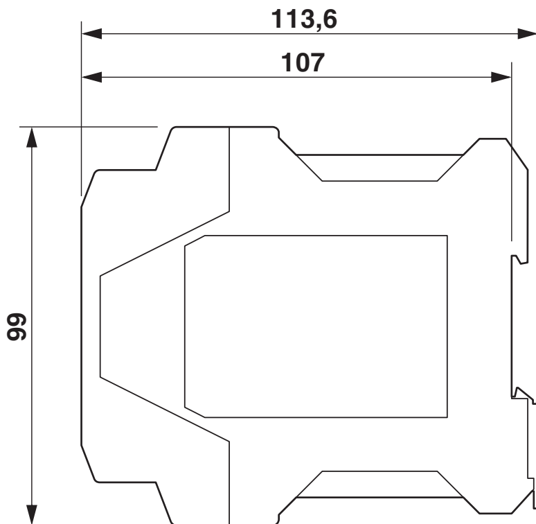
Maßzeichnung
