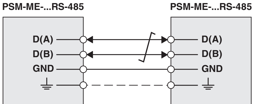
Anschlusszeichnung
