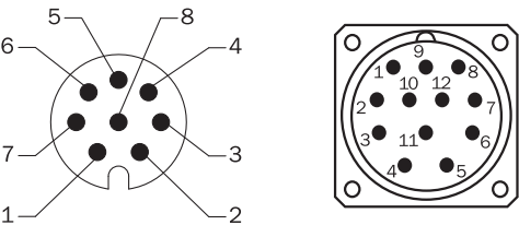
連至電纜線/外殼的M12 / M23設備公接頭視圖
