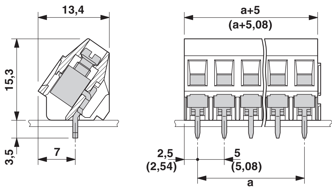
尺寸图
