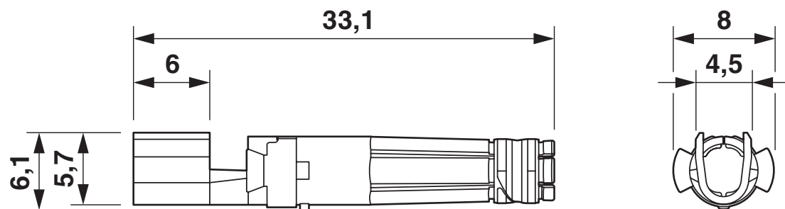
外形寸法
