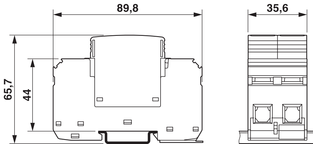
尺寸图
