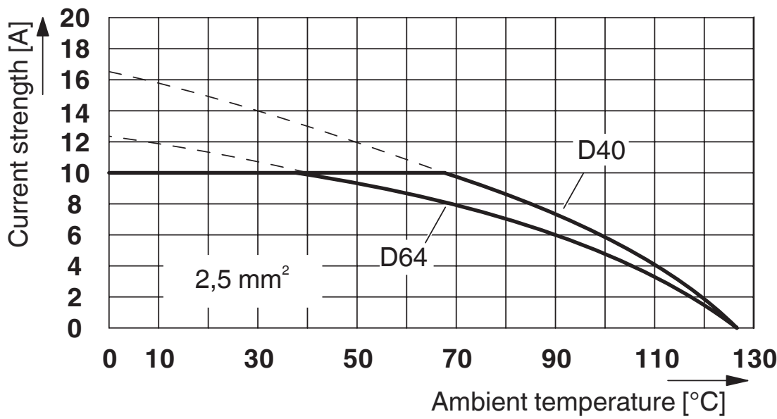
2.5 mm²的衰减曲线图
