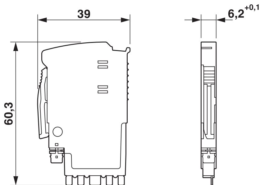
尺寸图
