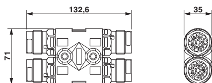
Maßzeichnung
