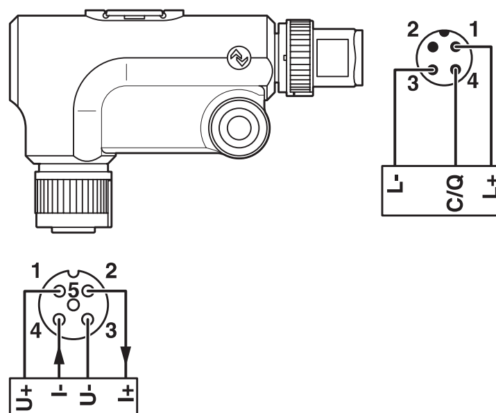
接线图
