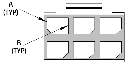
RECEPTACLE 43025
