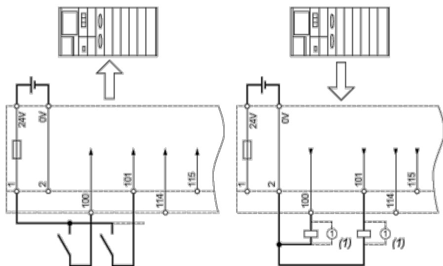
接线图
