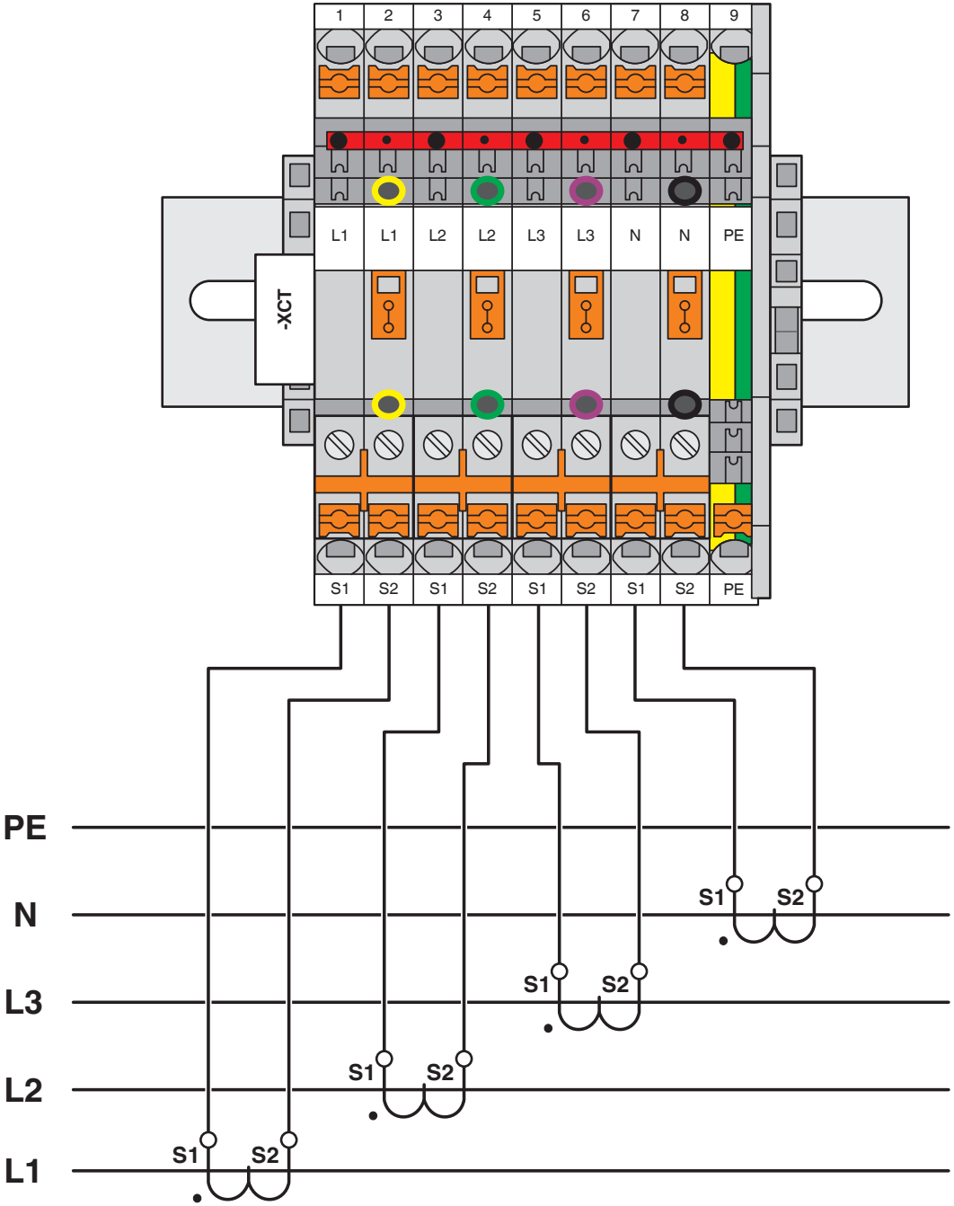
电路图
