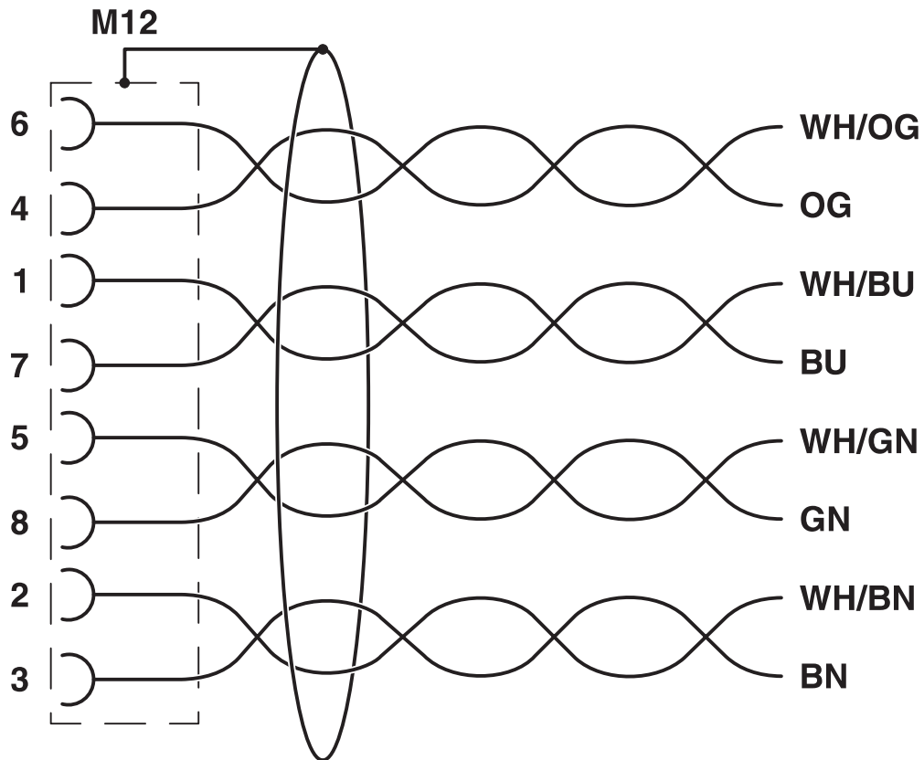
电路图
