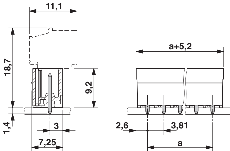
尺寸图
