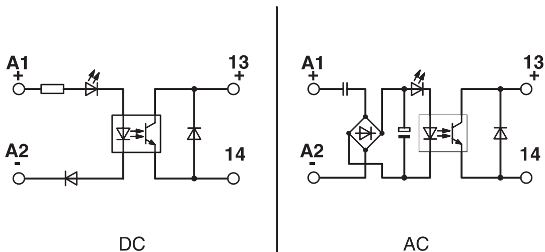
电路图
