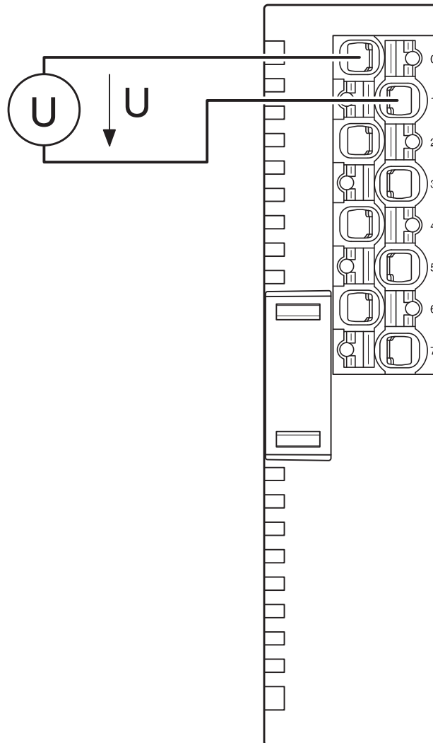
接线图
