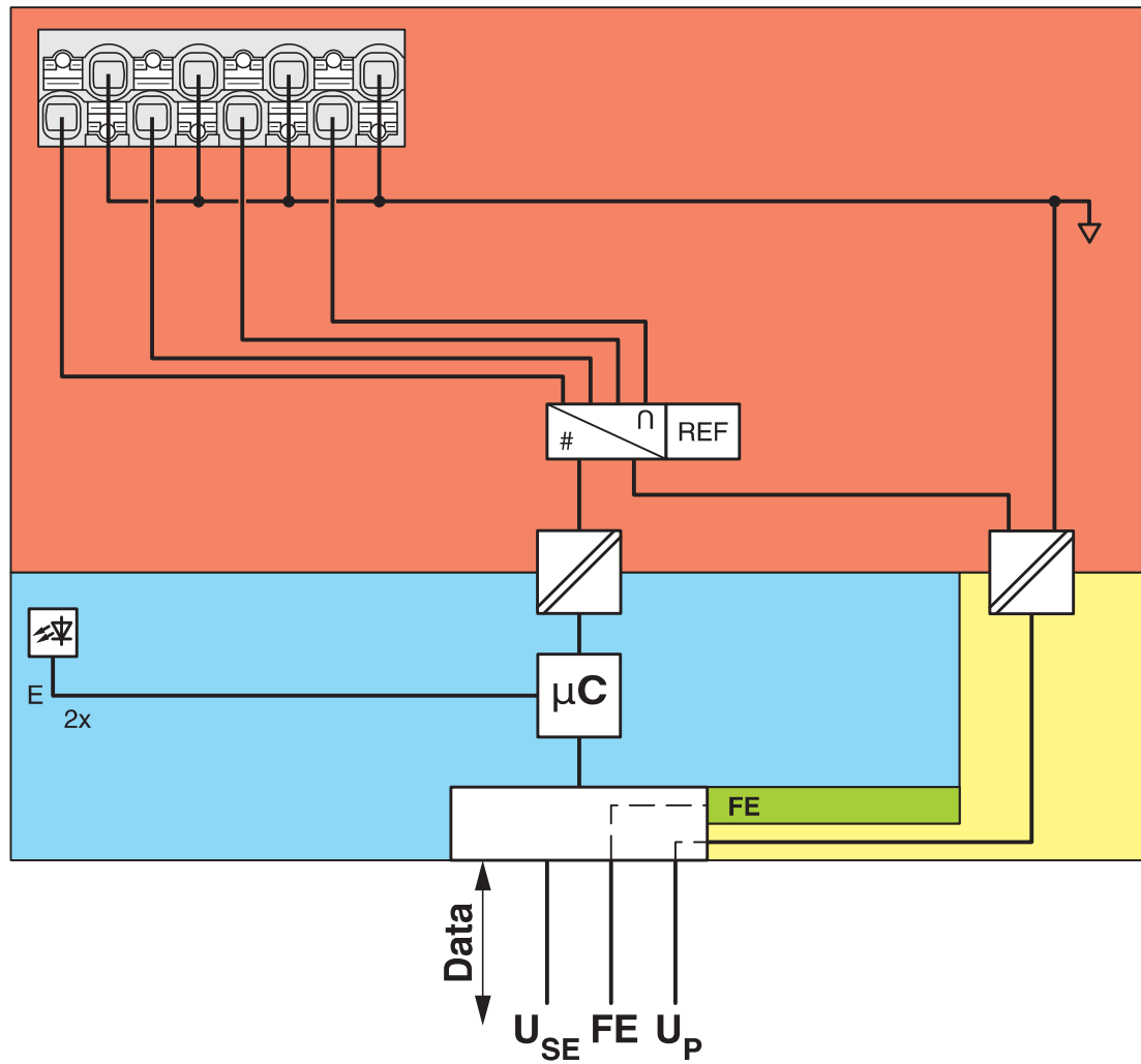
结构框图
