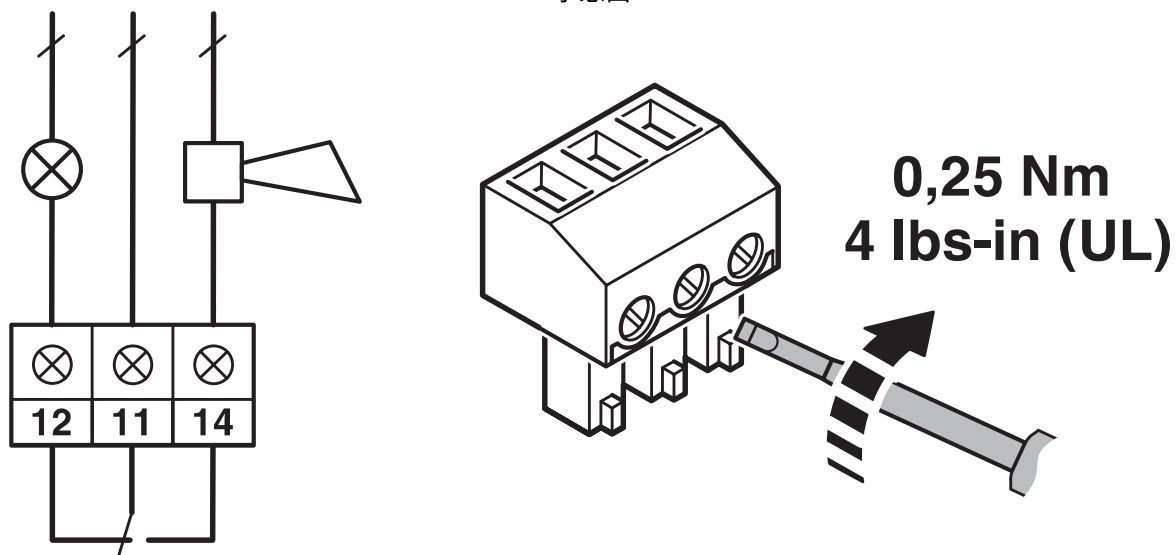
电涌保护器的遥信触点连接
