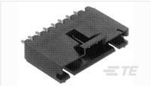
TE製品番号:5-103908-7 08 MTE HDR SRST LATCH W/HLDWN
