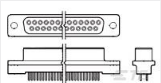
TE製品番号:5-103908-4 05 MTE HDR SRST LATCH W/HLDWN
