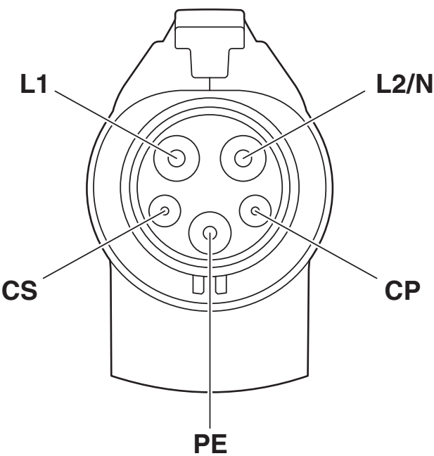
接线图
