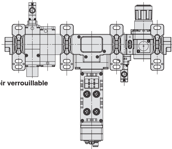
Côté arrière
