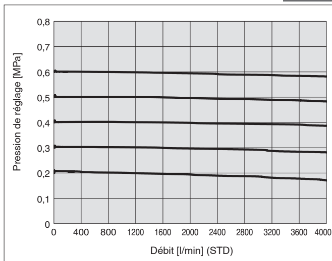
Pression d'alimentation 0.7 MPa
