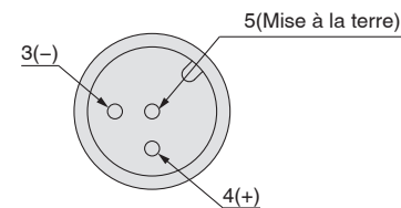
Figure détaillée de la section a du connecteur M12
