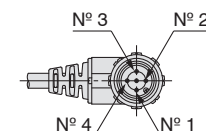
Disposition des broches du connecteur mâle
