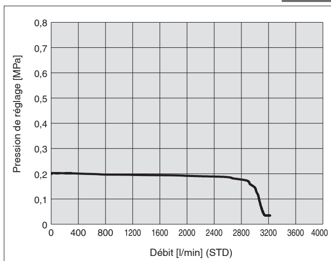
Pression d'alimentation 0.3 MPa
