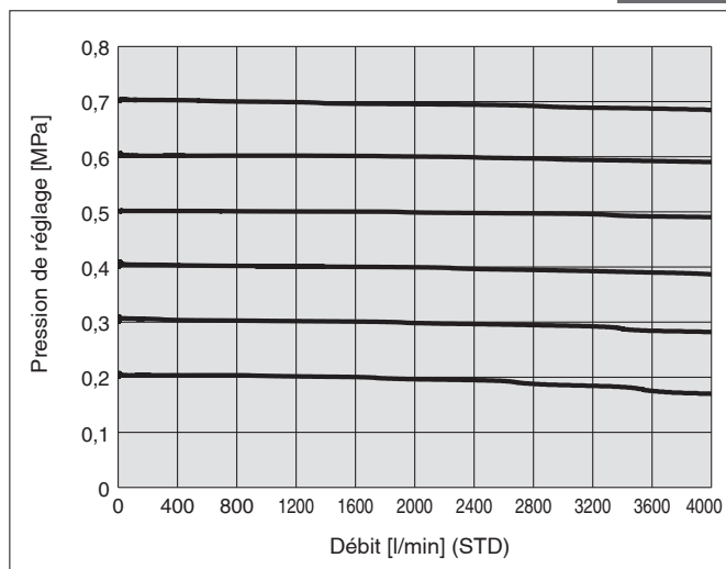
Pression d'alimentation 0.8 MPa
