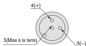
Figure détaillée de la section a du connecteur M12
