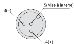
Figure détaillée de la section a du connecteur M12
