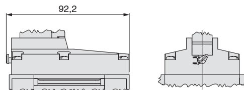
Détails de la partie commande manuelle (pour commande manuelle) Type E
