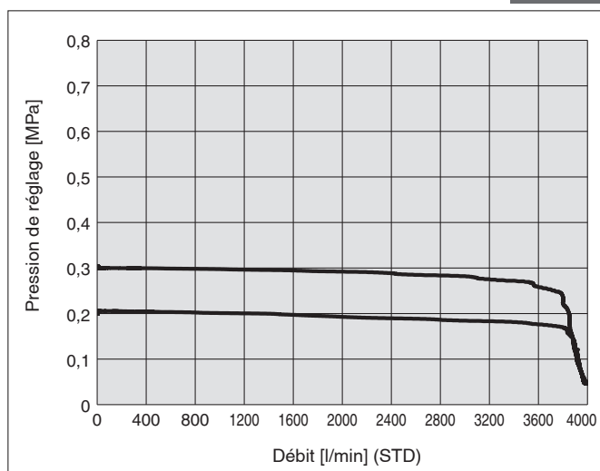
Pression d'alimentation 0.4 MPa
