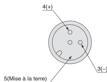
Figure détaillée de la section b du connecteur M12
