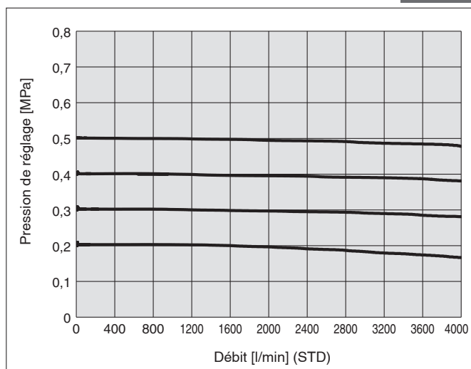
Pression d'alimentation 0.6 MPa
