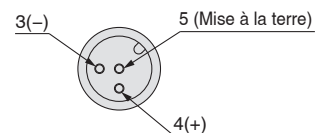
Figure détaillée de la section a du connecteur M12
