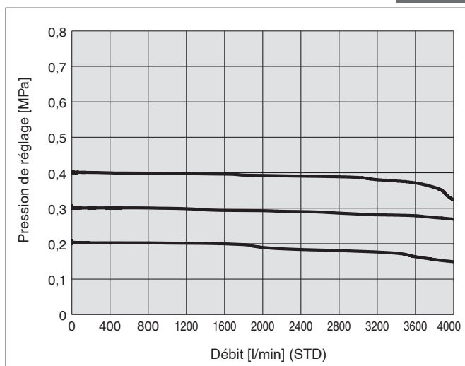
Pression d'alimentation 0.5 MPa
