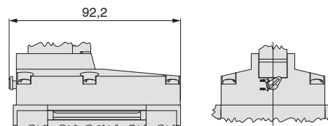
Détails de la partie commande manuelle (pour commande manuelle) Type E
