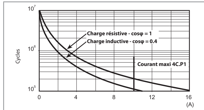
F 4C - Durée de vie électrique (AC) en fonction de la charge Types 4C.01/P1
