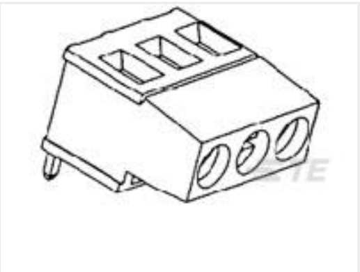
TE Part #282851-3 TERMI-BLOK PCB MOUNT 180 3P.5
