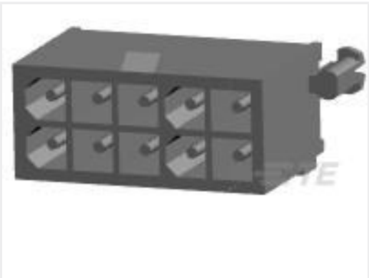
TE Part #1-770858-0 10P MINI UMN L HDR ASSY SNDBL L
