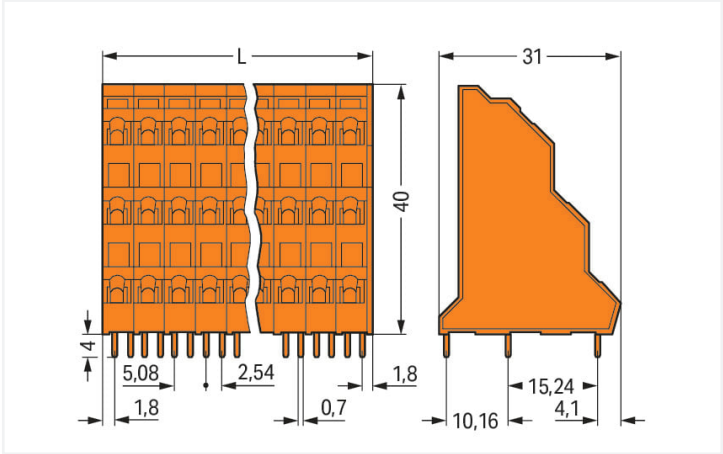
Dimensions en mm L = ((\text{nombre de pôles} / 3) \times \text{pas}) + 1 \text{ mm}
