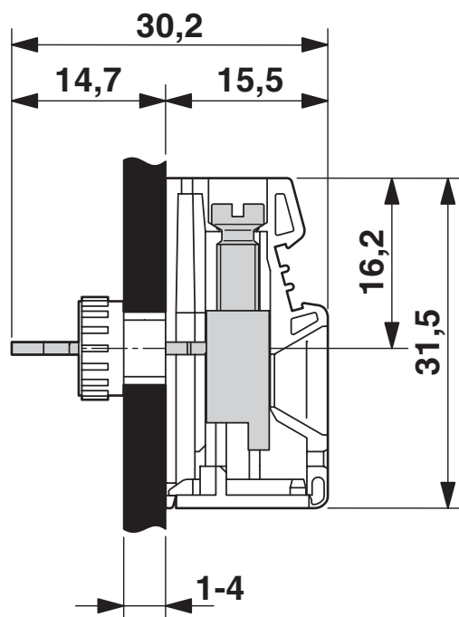
尺寸图
