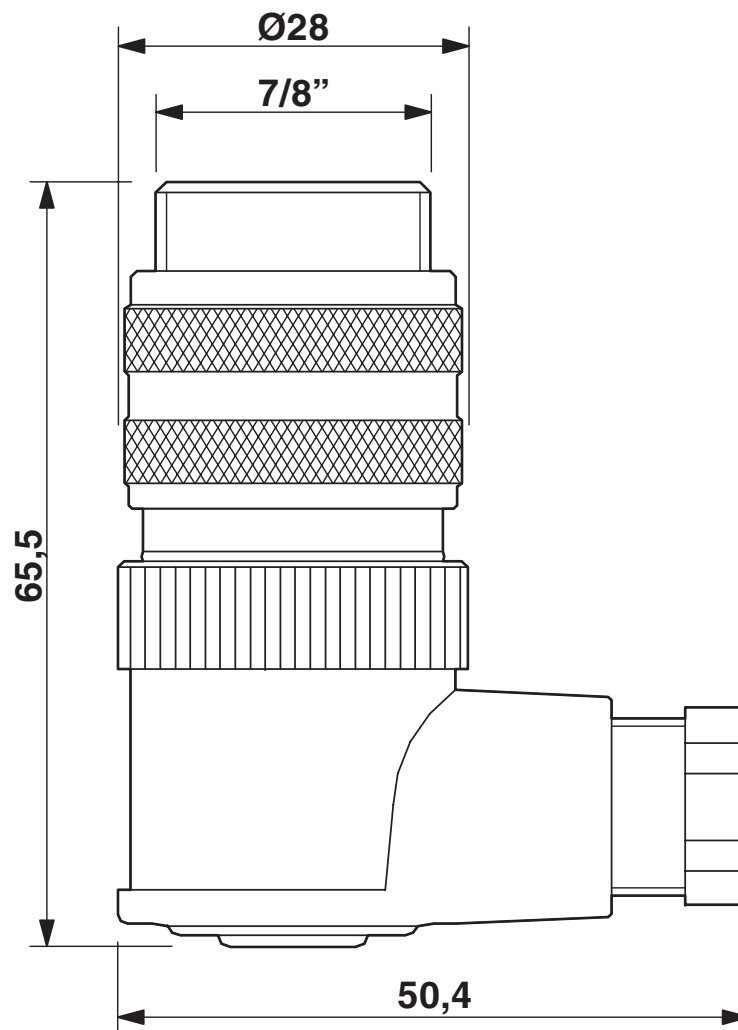
尺寸图
