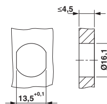
Maßzeichnung
