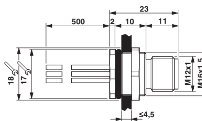
Maßzeichnung
