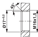
Maßzeichnung
