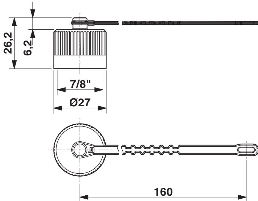
尺寸图
