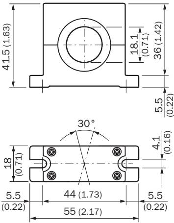
尺寸圖 (尺寸 (mm))
