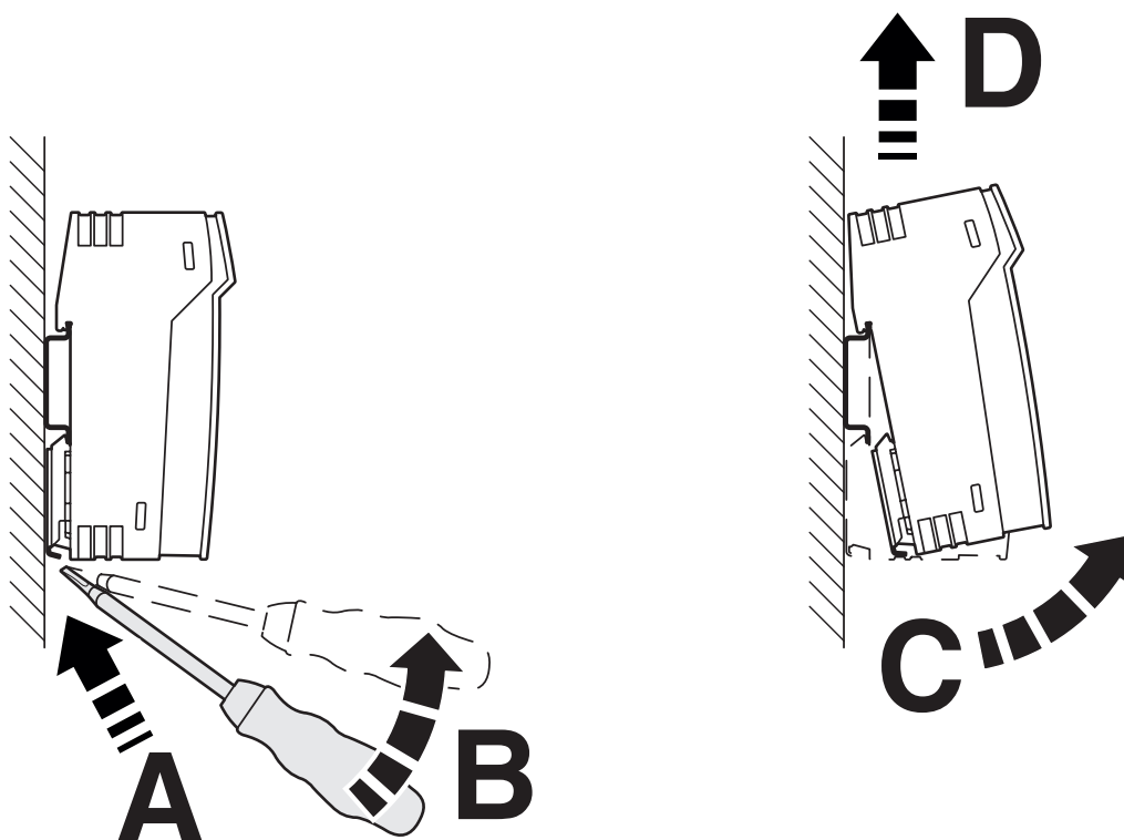
Schemazeichnung
