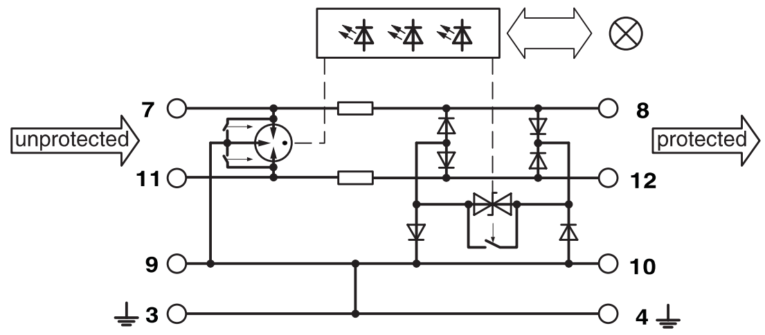
电路图
