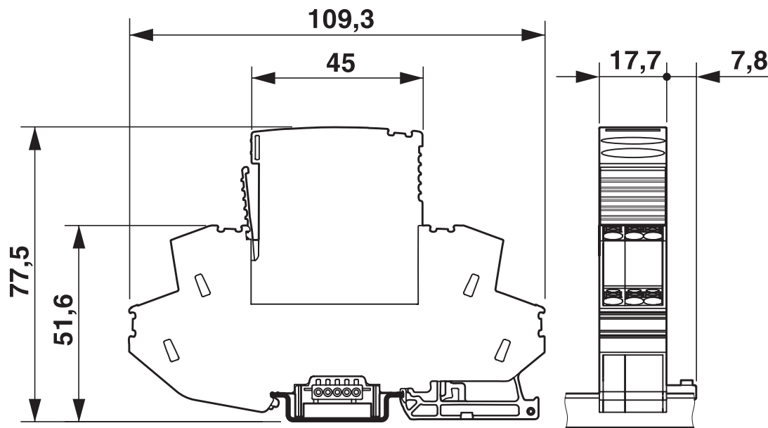
尺寸图
