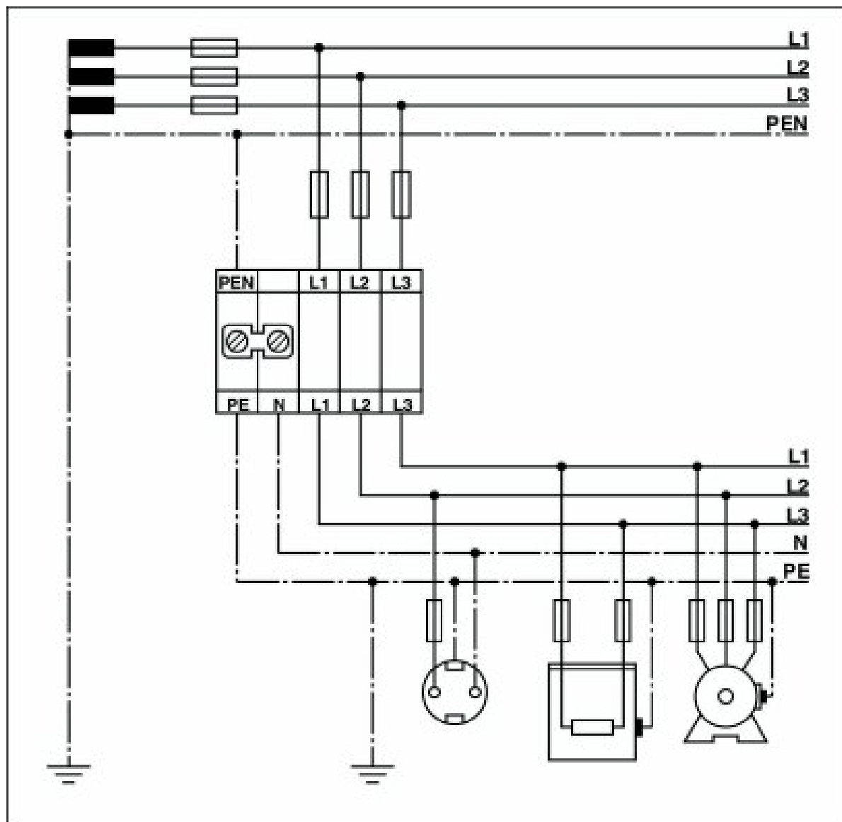
接线图
