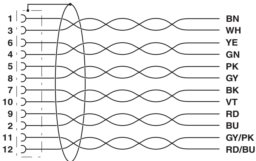
Kontaktbelegung der M12-Buchse
