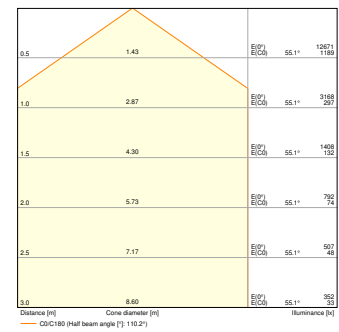
BATTEN CBO 1800 V 65W MS 840 WT
