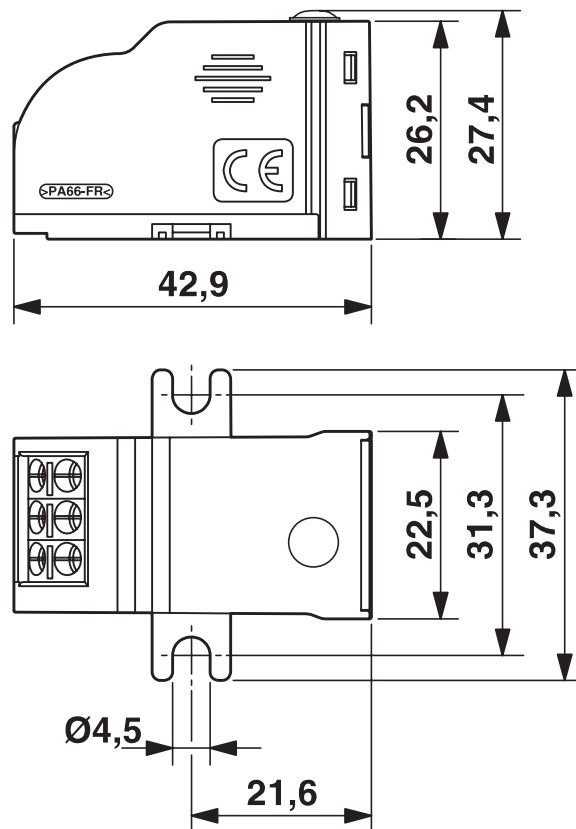
尺寸图
