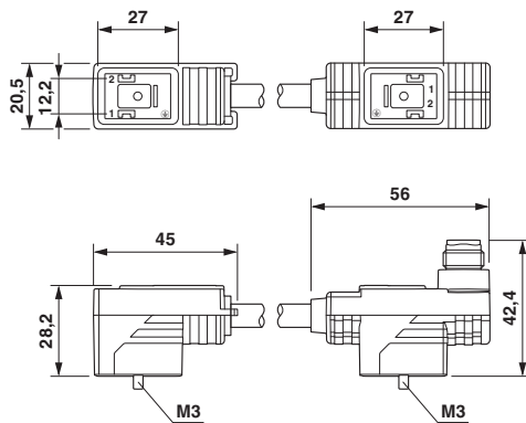
外形寸法
