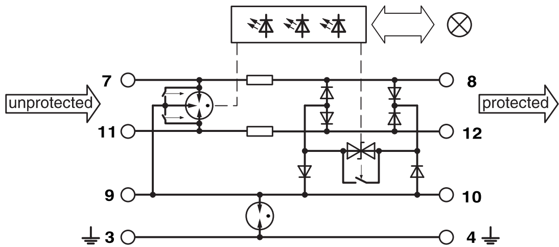
电路图
