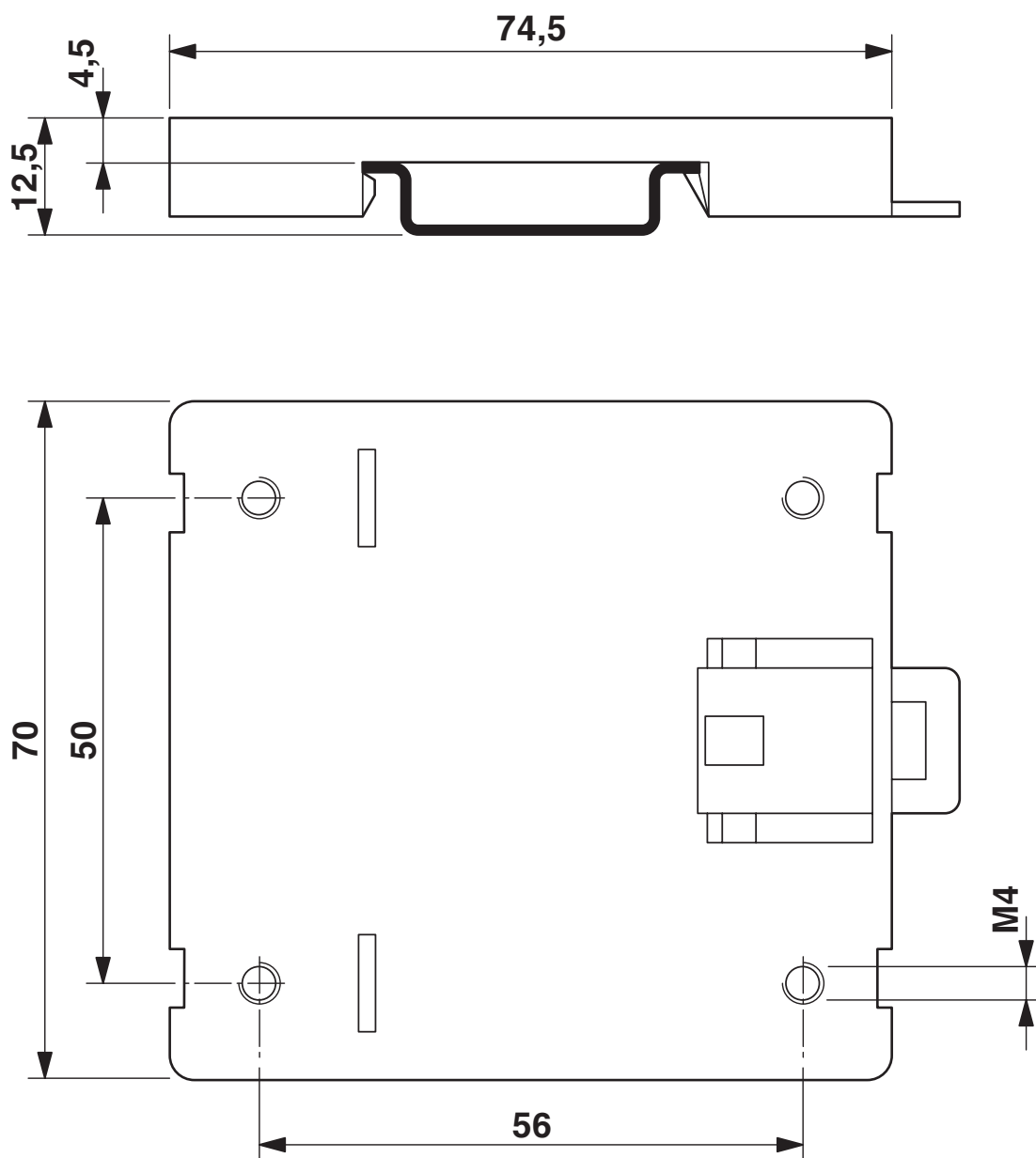
尺寸图
