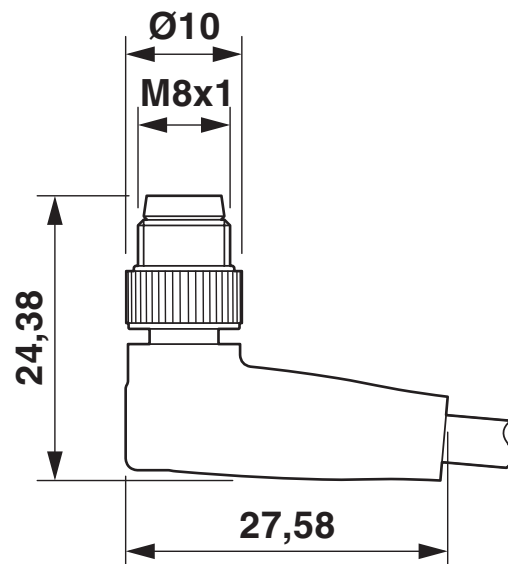
尺寸图
