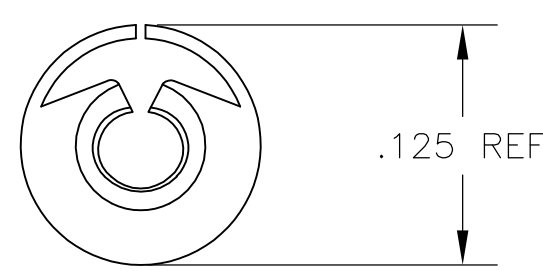
LOOSE PIECE -1,-3,-4,-6, & -8 ONLY
