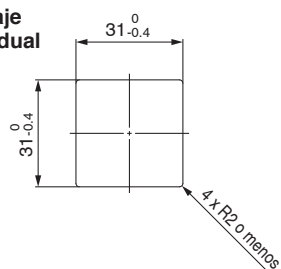
Montaje seguro múltiple (2 uds. o más) <Horizontal>
