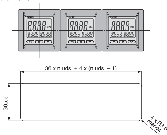
Montaje seguro múltiple (2 uds. o más) <Horizontal>
