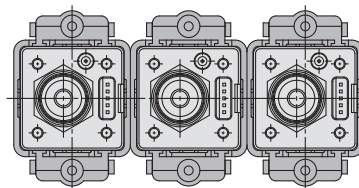
Ejemplo de montaje en panel <Horizontal>
