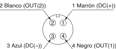
Asignación de pins del conector
