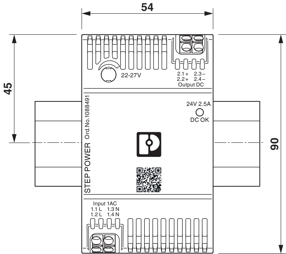
尺寸图
